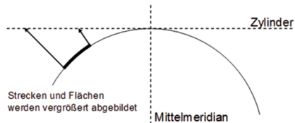
Abb. 9: Gauß-Krüger-Abbildung
