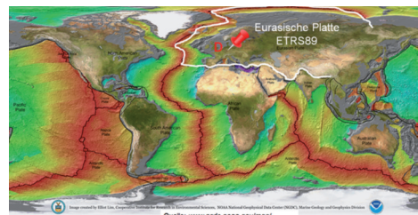
Abb. 5: Kontinentalplatten geozentrisches Koordinatensystem
