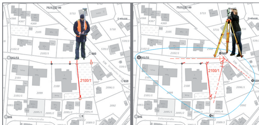
Abb. 29: exemplarische Vorgehensweise nach der Umstellung auf ETRS89/UTM bei Katastervermessungen in Gemarkungen mit Vollzugserklärung (links: SAPoS®-Verfahren, rechts: Polarverfahren)
